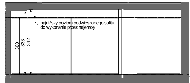
PRZEKRÓJ "A-A" PRZEZ LOKAL USŁUGOWY
