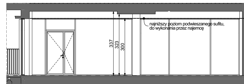
PRZEKRÓJ "A-A" PRZEZ LOKAL USŁUGOWY
